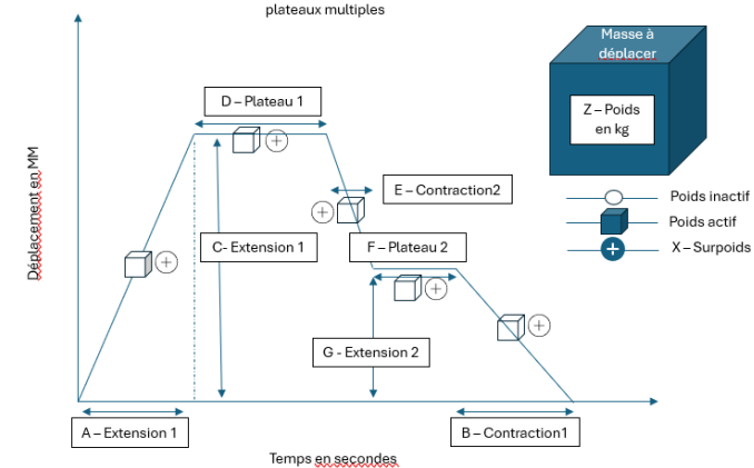
TYPE 3 - Mouvement avec plateaux multiples
